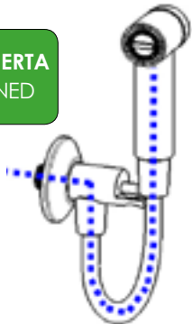
AVVICINARE LA CALOTTA DELLA DOCCIA ALLA VALVOLA PLACE THE SHOWER CAP NEAR THE SHUT-OFF VALVE
